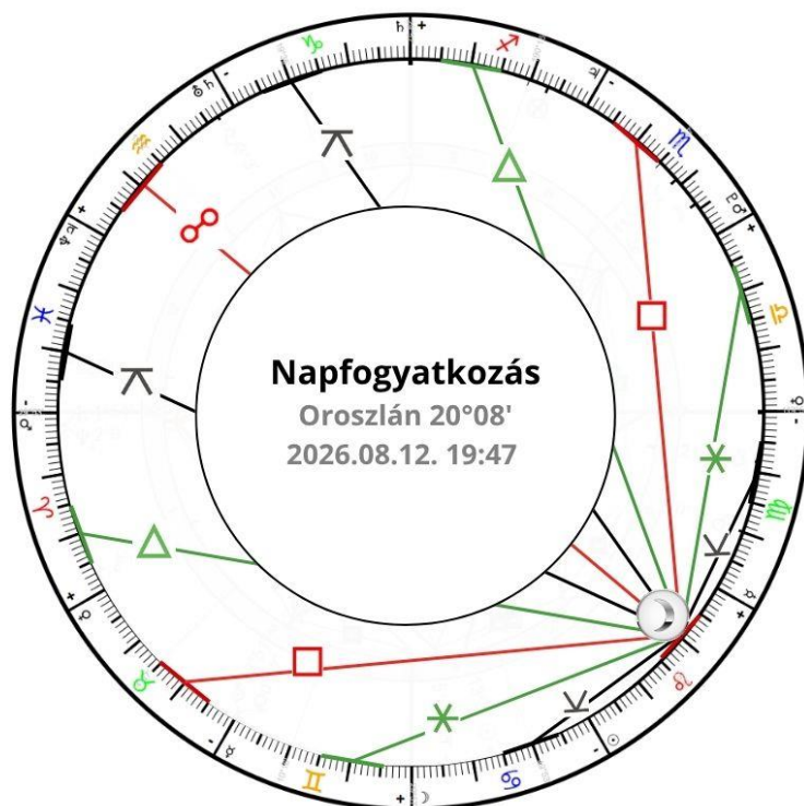
17. ábra: Napfogyatkozás hatása (2026.08.12. 19:47 Bp.)
