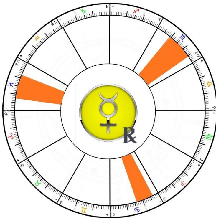
21. ábra: Retrográd Merkúr hatása
