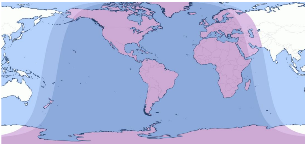
18. ábra: Holdfogyatkozás térkép (2026.08.28.)
