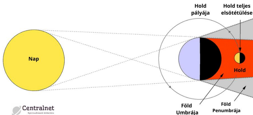
8. ábra: Teljes Holdfogyatkozás geometriája
