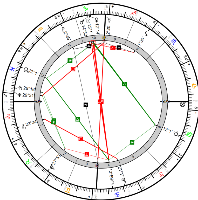
30. ábra: Rák Telihold (2026.01.03. 11:02 Bp.)
