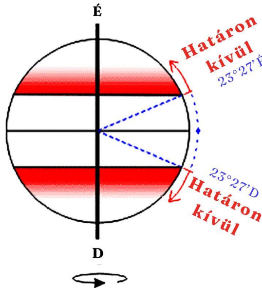
7. ábra: Határon kívüli deklináció
